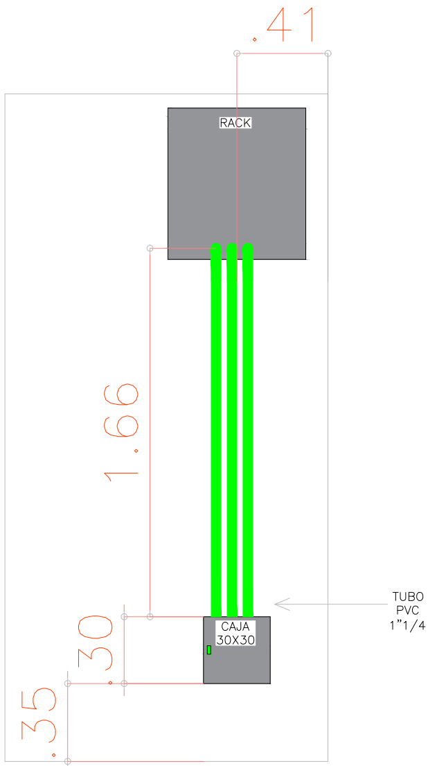
DETALLE RACK ESC. S/N
