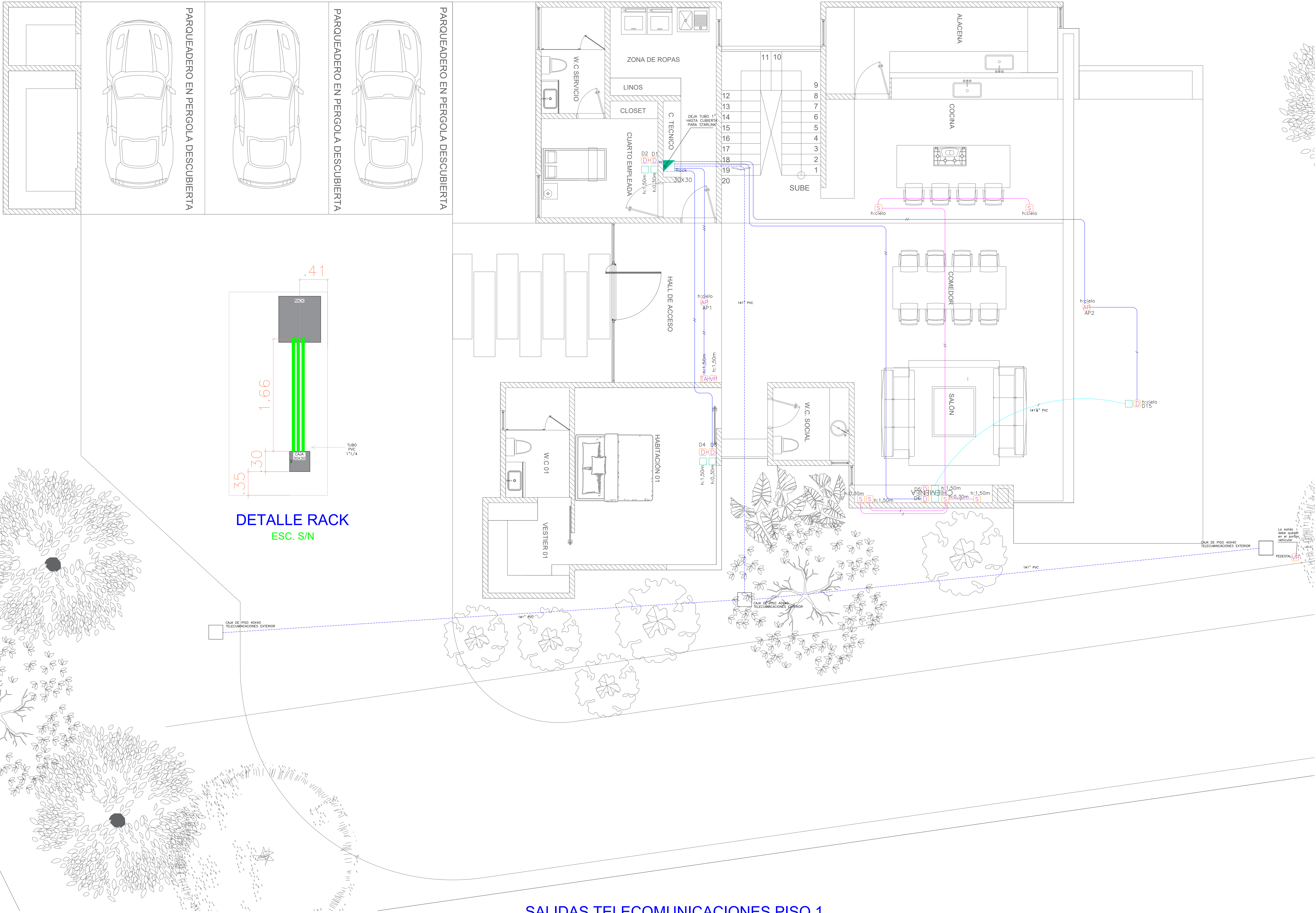
SALIDAS TELECOMUNICACIONES PISO 1 ESC. S/N
